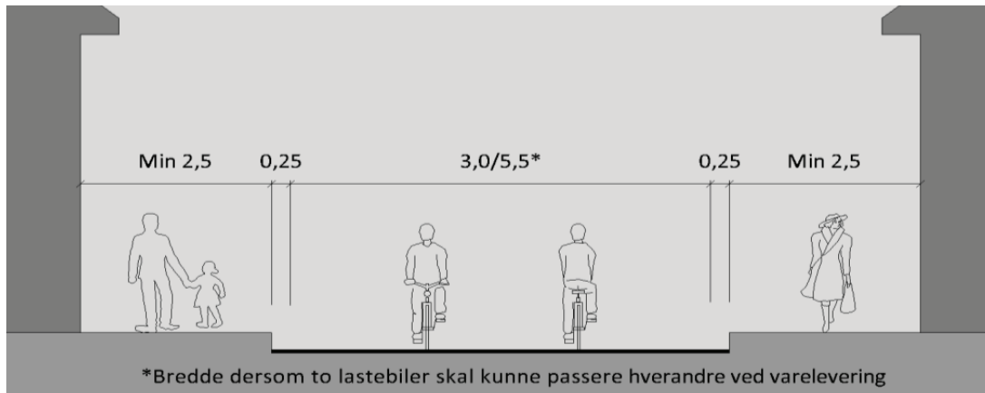
Figur 3.12: Utforming av sykkelgate (mål i m)
