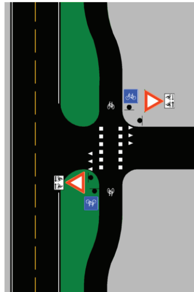
Figur 4.14: Kryssing mellom veg og sykkelveg der kryssende trafikk på sekundærvegen skal vike for syklende
