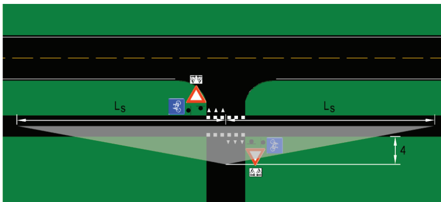
Figur 4.26: Sikt mellom gang- og sykkelveg / sykkelveg og veg der trafikken på vegen har vikeplikt (mål i m)
