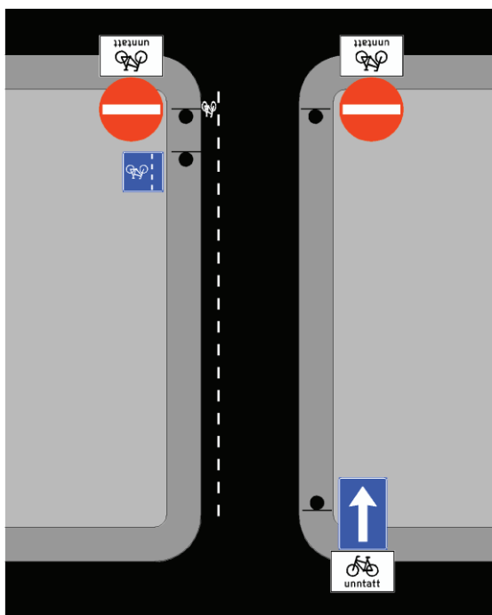
Figur 3.16: Skilting og oppmerking i envegsregulerte gater når sykling mot kjøreretningen tillates. Sykkelfelt mot kjøreretningen og blandet trafikk med kjøreretningen.
