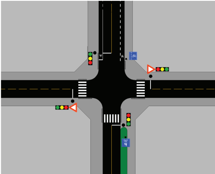
Figur 4.21: Systemskifte gang- og sykkelveg og sykkelfelt
