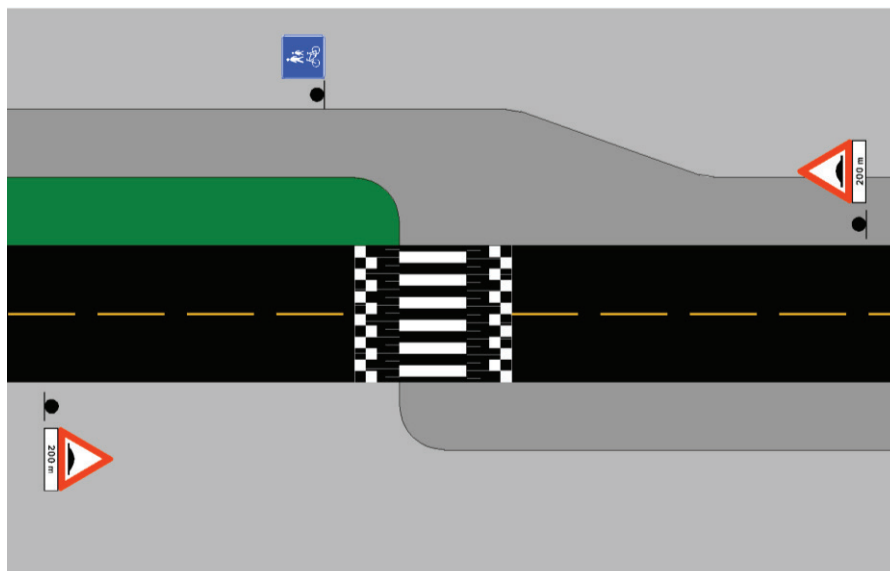
Figur 3.18: Systemskifte mellom blandet trafikk og gang- og sykkelveg
