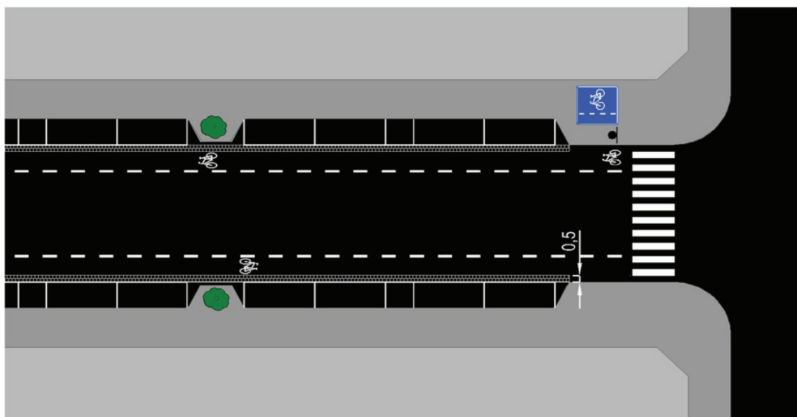
Figur 3.7: Eksempel på sykkelfelt kombinert med kantparkering (mål i m)
