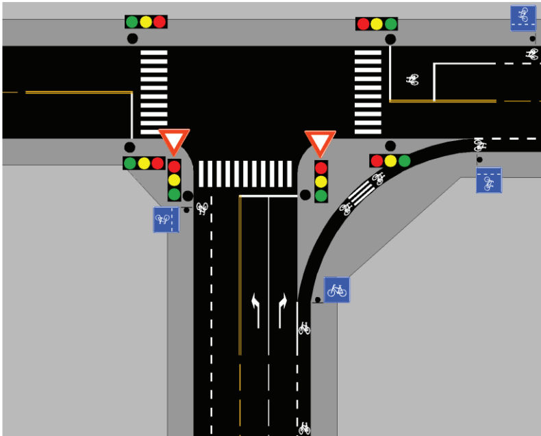
Figur 4.10: Eksempel på filterfelt for syklende
