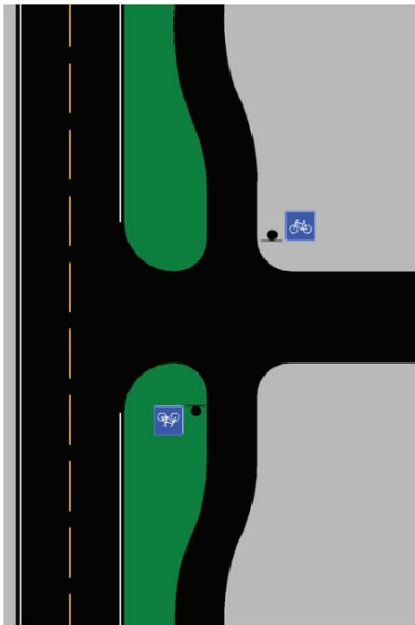
Figur 4.13: Kryssing mellom veg og sykkelveg der syklende fra sykkelveg skal vike for trafikk på veg
