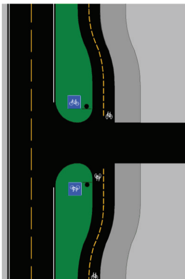
Figur 4.15: Kryssing mellom veg og sykkelveg med fortau der syklende fra sykkelveg har vikeplikt
