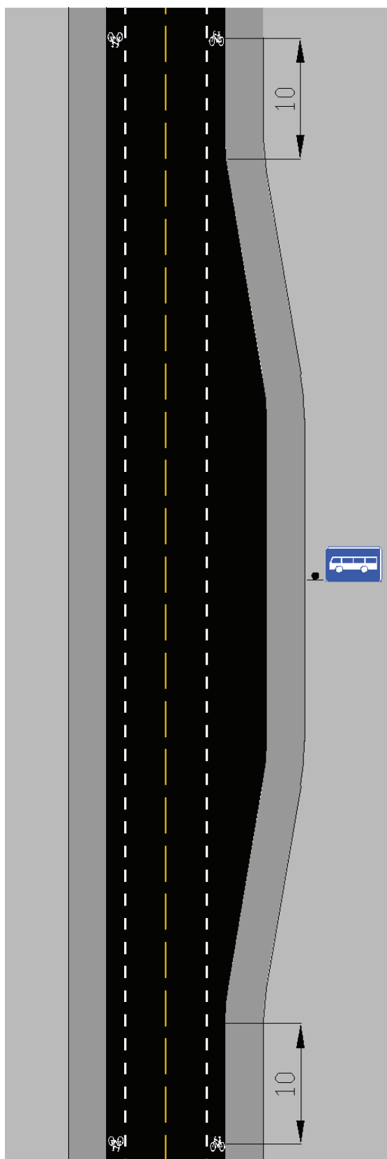
Figur 3.4: Sykkelfelt til venstre for busslomme
