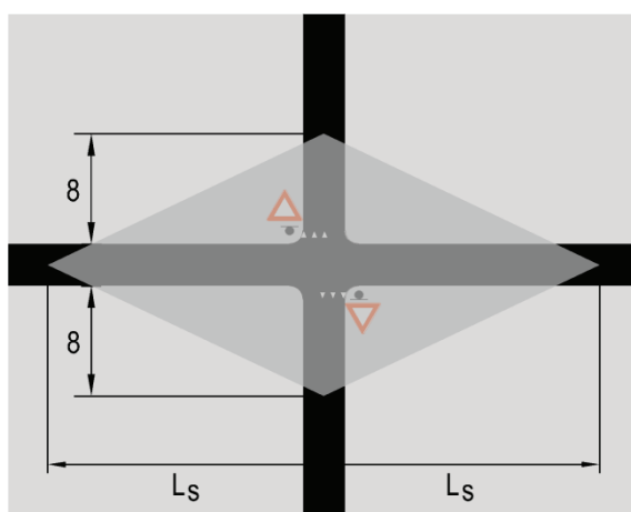
Figur 4.28: Siktkrav mellom to kryssende gang- og sykkelveger / sykkelveger med vikepliktsregulering på en av vegene (mål i m)
