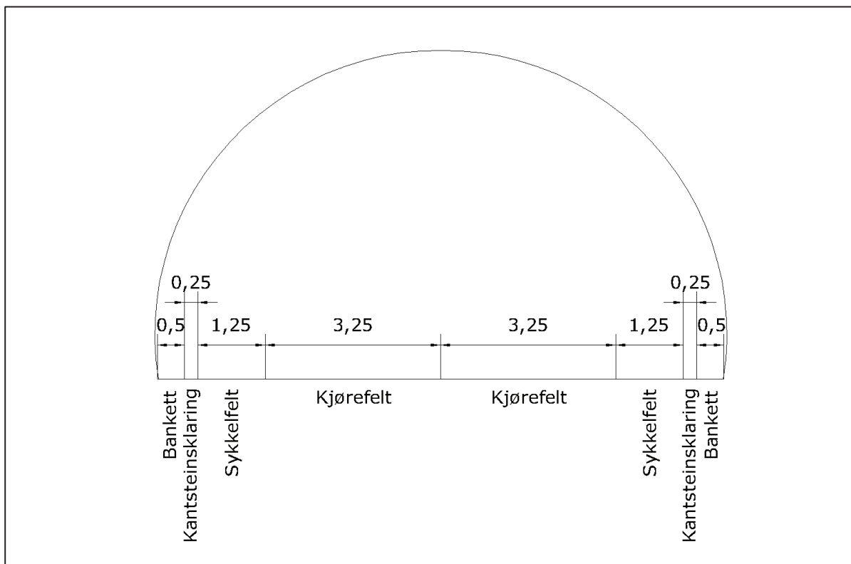
Tunnelprofil T10,5 SF: To kjørefelt og sykkelfelt
