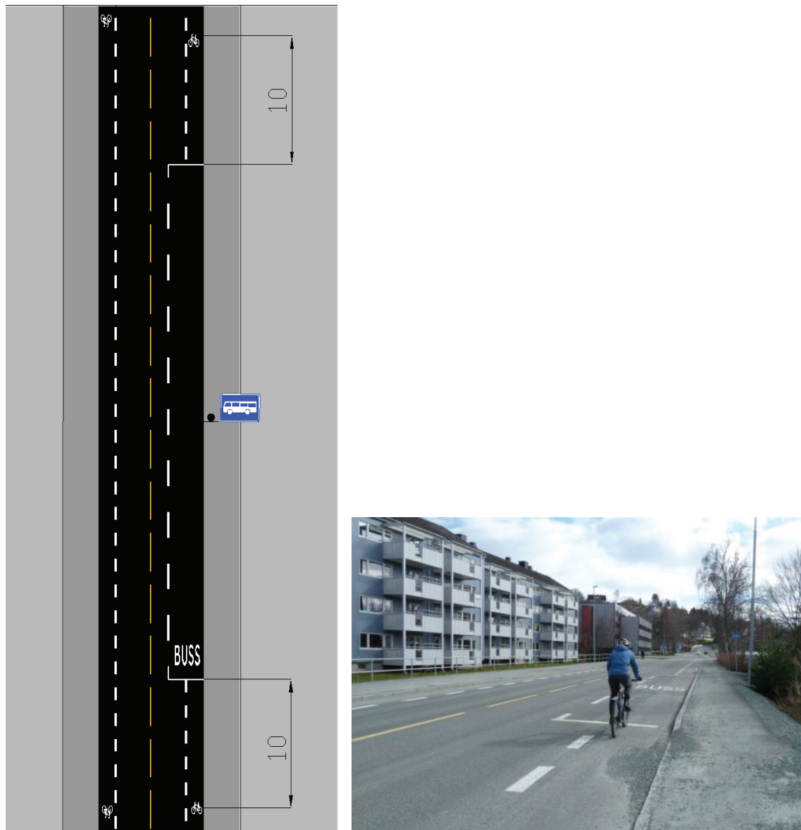
Figur 3.6: Sykkelfelt på strekning med kantstopp for buss
