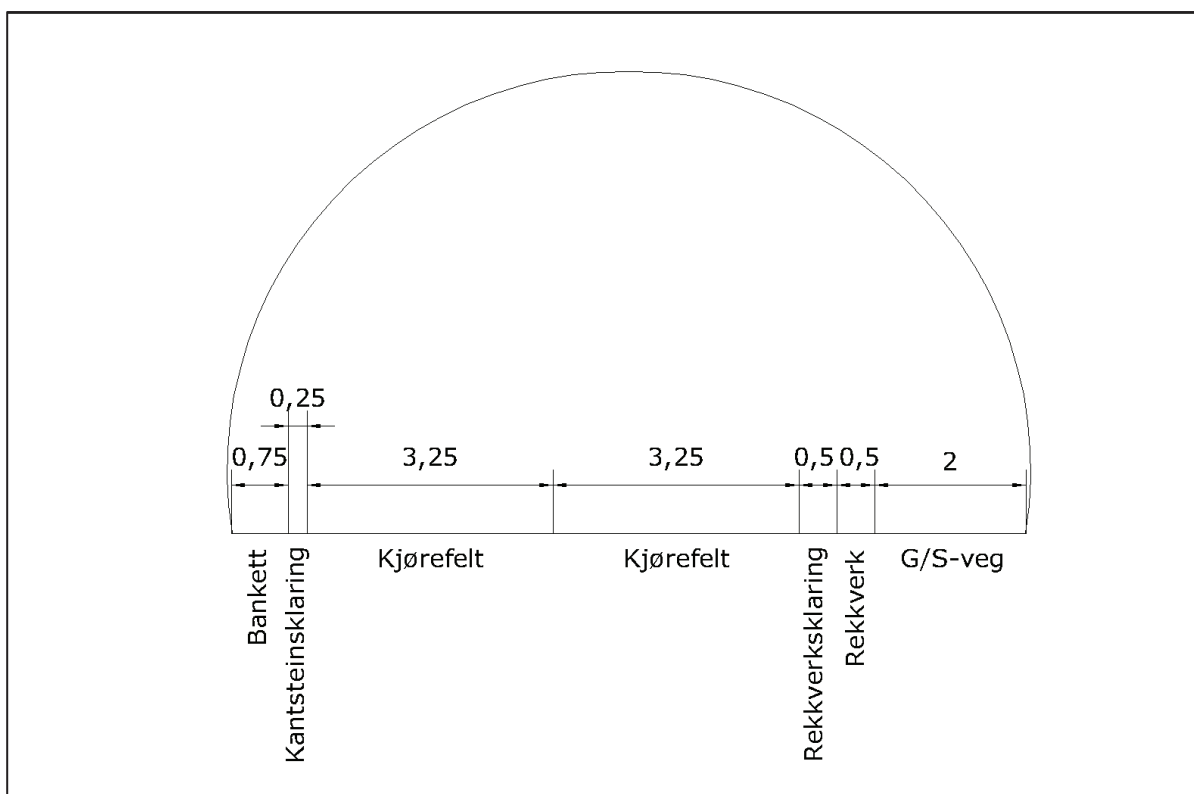
Tunnelprofil T10,5 GS: To kjørefelt, gang- og sykkelveg adskilt med rekkverk
