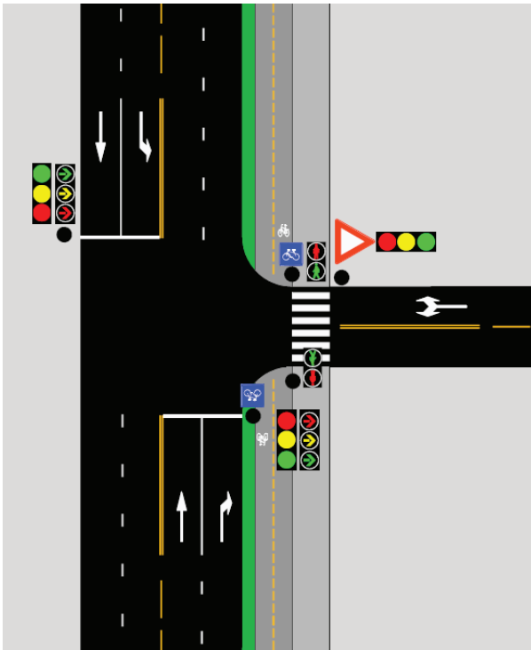
Figur 4.18: Signalregulert kryss som er vikepliktsregulert når signalene er ute av drift.
