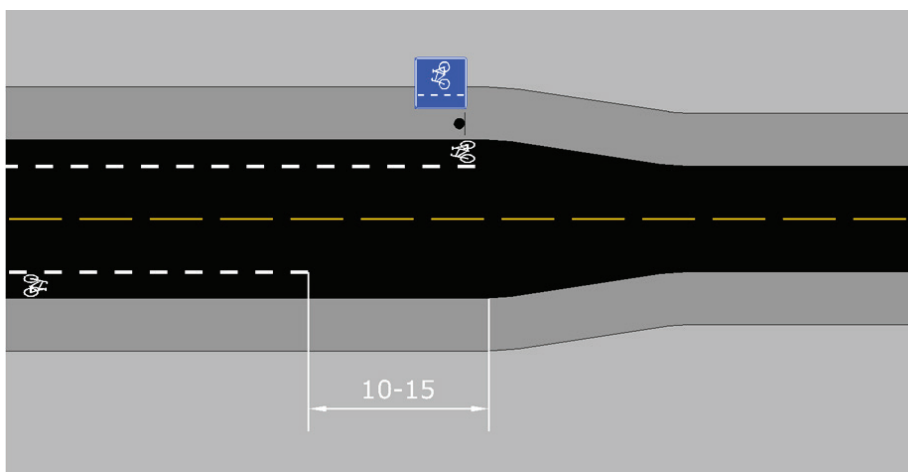
Figur 3.19: Systemskifte mellom blandet trafikk og sykkelfelt (mål i m)
