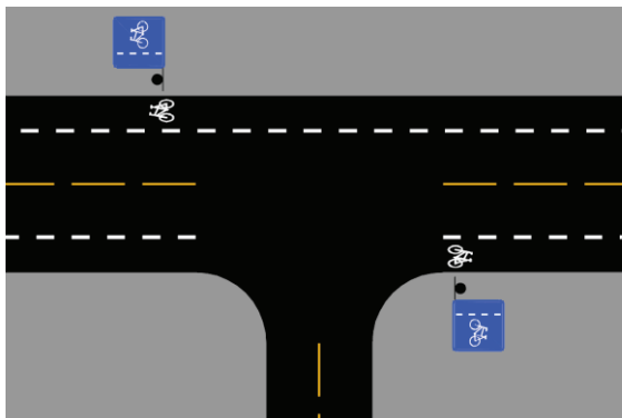
Figur 4.3: Skilting og oppmerking av sykkelfelt i høyreregulert T-kryss
