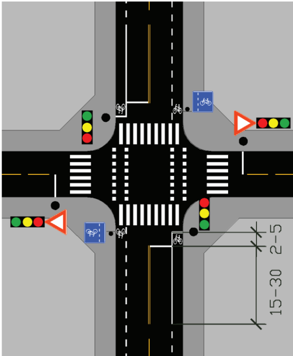
Figur 4.7: Tilbaketrukket stoplinje for motorvogn i signalregulert kryss (mål i m)
