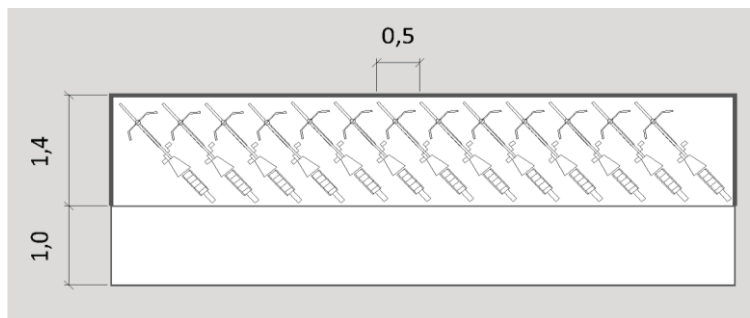
Figur 5.2: Dimensjonering av sykkelparkering, skrå (mål i m)
