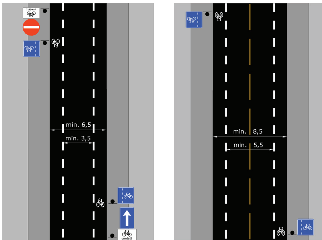
Figur 3.3 Minimum veg- og kjørefeltbredde ved oppmerking av sykkelfelt i gate med henholdsvis ett kjørefelt (envegsregulert) og to kjørefelt
