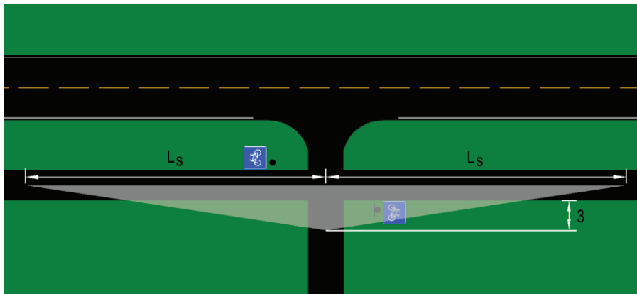
Figur 4.25: Sikt mellom gang- og sykkelveg / sykkelveg og avkjørsel (mål i m)
