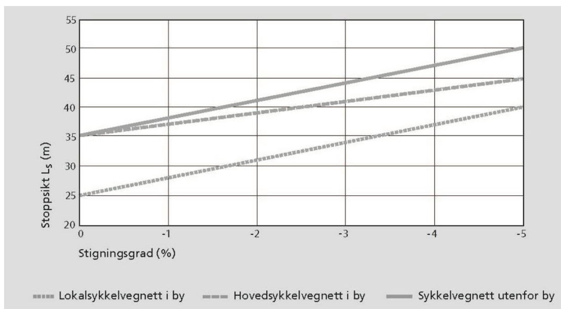
Figur 4.23: Stoppsikt ( L_s ) for syklende avhengig av type nett, omgivelser og stigningsgrad
