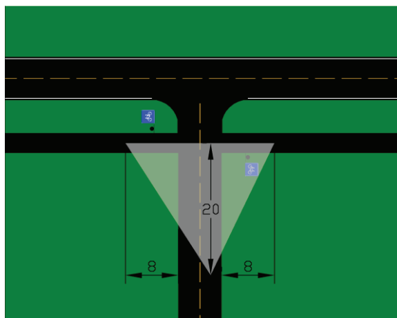
Figur 4.24: Sikt mellom gang- og sykkelveg / sykkelveg med fortau og veg der syklende har vikeplikt (mål i m)
