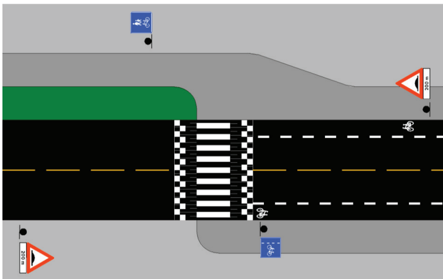
Figur 3.20: Systemskifte mellom gang- og sykkelveg og sykkelfelt
