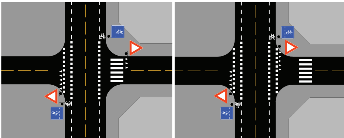
Figur 4.5: Skilting og oppmerking av sykkelfelt i forkjørsregulert kryss med gangfelt, henholdsvis nær krysset (til venstre) og med gangfeltet trukket tilbake fra krysset (til høyre)
