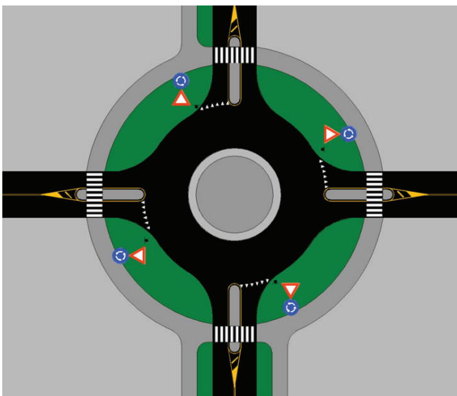
Figur 4.20: Gang- og sykkelveg i rundkjøring
