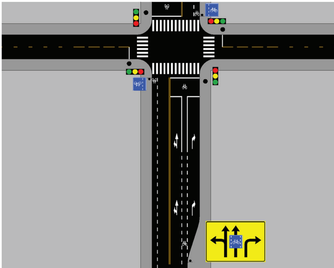
Figur 4.9: Midtstilt sykkelfelt
