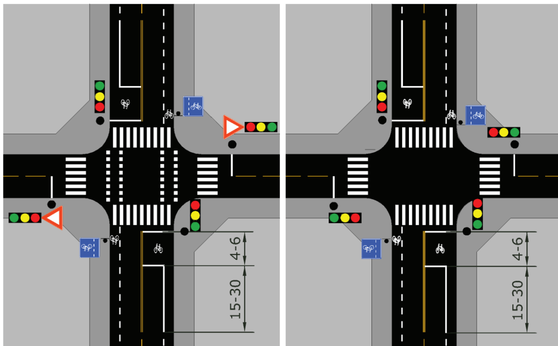
Figur 4.6: Skilting og oppmerking av sykkelfelt, hhv med og uten sykkelkryssing gjennom signalregulerte kryss (mål i m)
