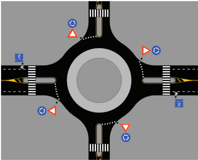
Figur 4.19: Rundkjøring med blandet trafikk og sykkelfelt i tilfartene.
