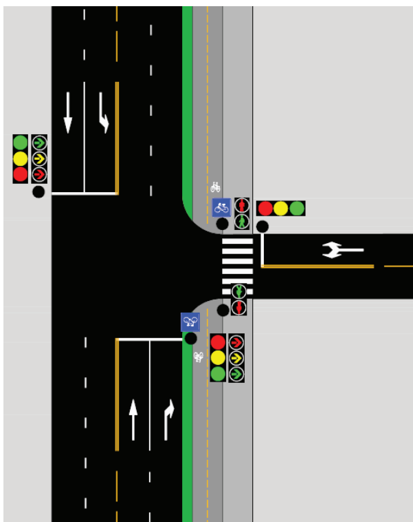
Figur 4.17: Signalregulert kryss som er uregulert når signalene er ute av drift.
