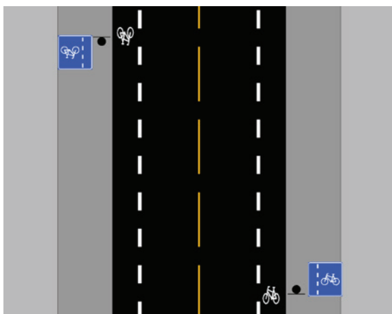
Figur 3.2 Skilting og oppmerking av sykkelfelt
