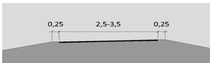
Figur 3.9: Tverrprofil for gang- og sykkelveg (mål i m)
