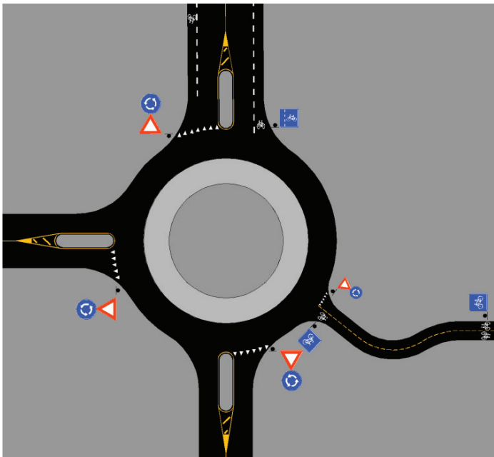
Figur 4.22: Systemskifte i rundkjøring, sykkelveg og sykkelfelt/ blandet trafikk
