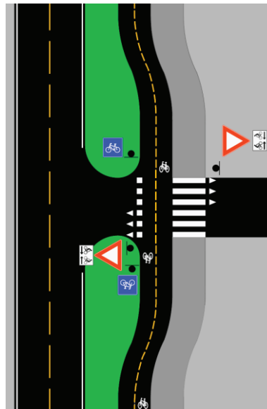
Figur 4.16: Kryssing mellom veg og sykkelveg med fortau der kryssende trafikk på sekundærvegen skal vike for syklende
