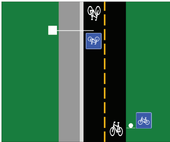
Figur 3.10: Skilting og oppmerking av sykkelveg med fortau
