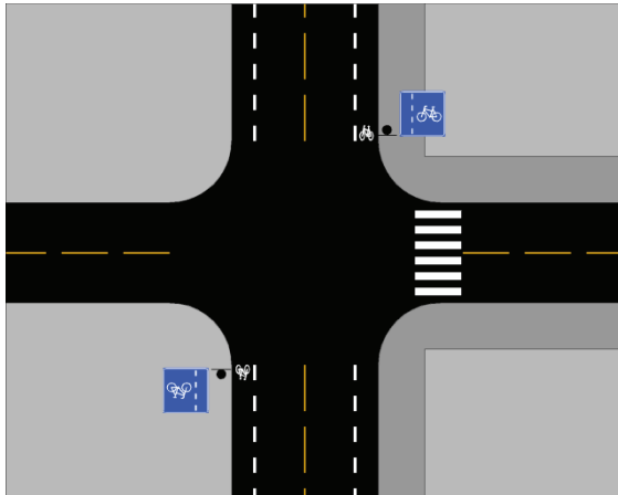
Figur 4.2: Skilting og oppmerking av sykkelfelt i høyreregulert X-kryss
