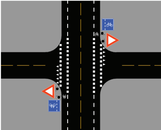
Figur 4.4: Skilting og oppmerking av sykkelfelt i forkjørsregulert kryss
