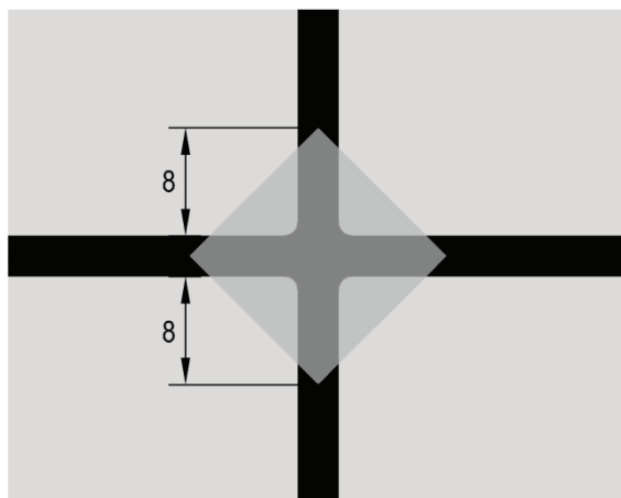
Figur 4.27: Sikt mellom to kryssende gang- og sykkelveger / sykkelveger i høyreregulert kryss (mål i m)
