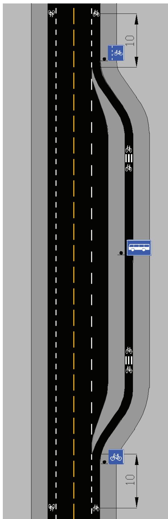
Figur 3.5: Sykkelveg til høyre for busslomme
