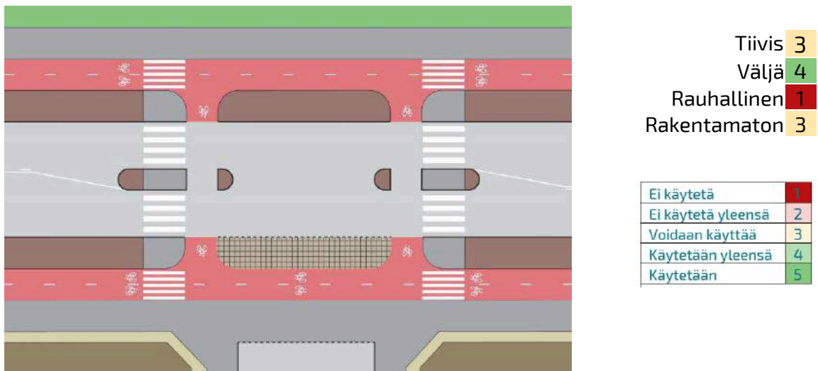
Kuva 141 Pyöräliikenteen kaksivaiheinen pääsuunnan ylitys. Pyöräliikenteen ryhmitysalue jaetaan suunnittain.
