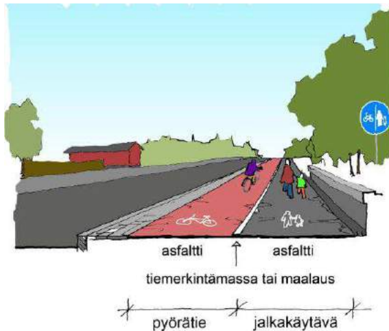
Kuva 35 Tiemerkintäerottelu.
