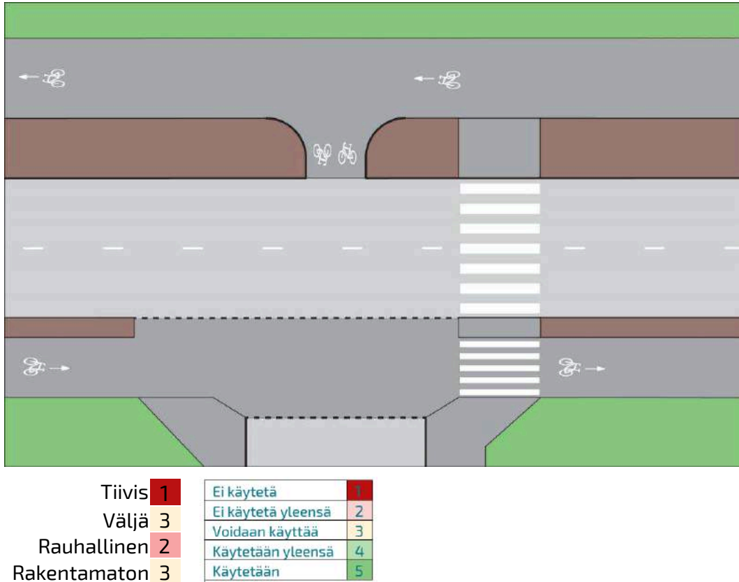
Kuva 122 Yksisuuntaisen pyörätien järjestely, jossa jalankulkijoiden käytössä ei ole jalkakäytävää.
