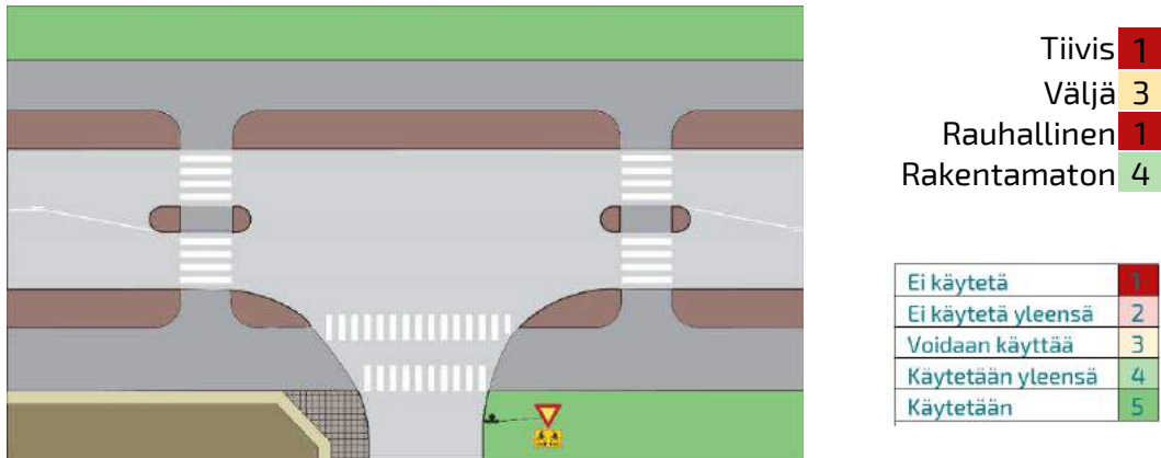
Kuva 144 Yhdistetyllä pyörätiellä ja jalkakäytävällä pääsuunta voidaan ylittää suojatietä pitkin. Risteävällä tiellä oleva jalkakäytävä erotellaan yhdistetystä pyörätiestä selkeästi.
