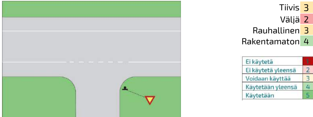
Kuva 109 Kylätie merkitään risteyksen kohdalla reunaviivan jatkeella ja sivusuunnat merkitään väistämisvelvollisiksi.
