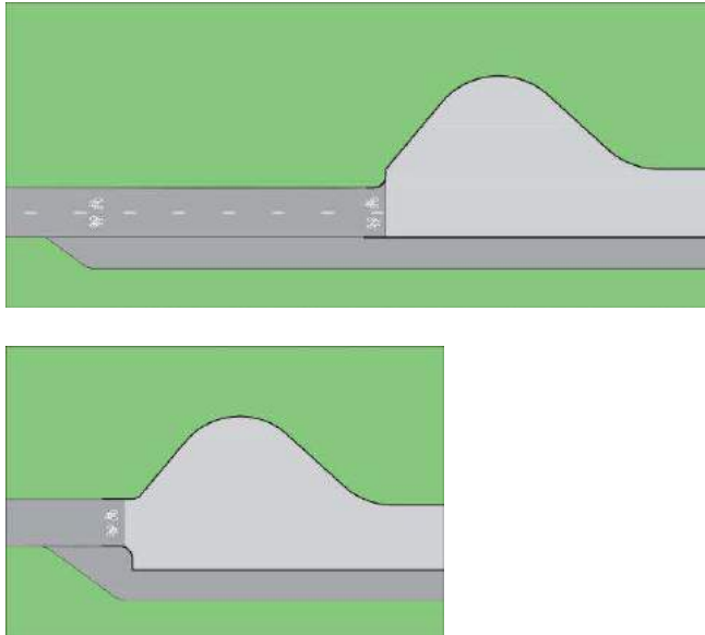
Kuva 159 Saumakohta päättyvän tien tai kadun kääntöpaikan kohdalla. Saumakohta toteutetaan vastaavalla tavalla myös ilman jalkakäytävää.
