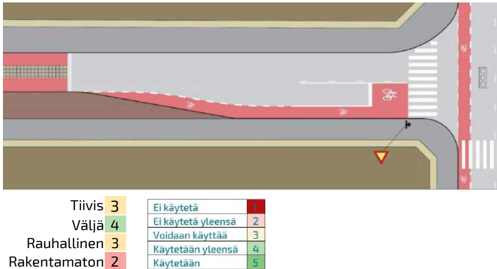
Kuva 130 Pyöräkadun normaali poikkileikkaus voidaan päättää 30–50 m ennen liikennevalo-ohjattua risteystä.
