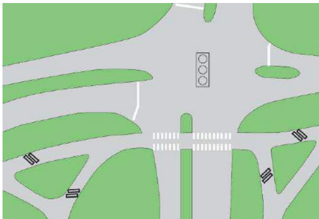
Kuva 169 Pyöräliikenteen pääreiteille järjestetty ilmaisualue vain liikennevaloihin tulevalle liikenteelle.
