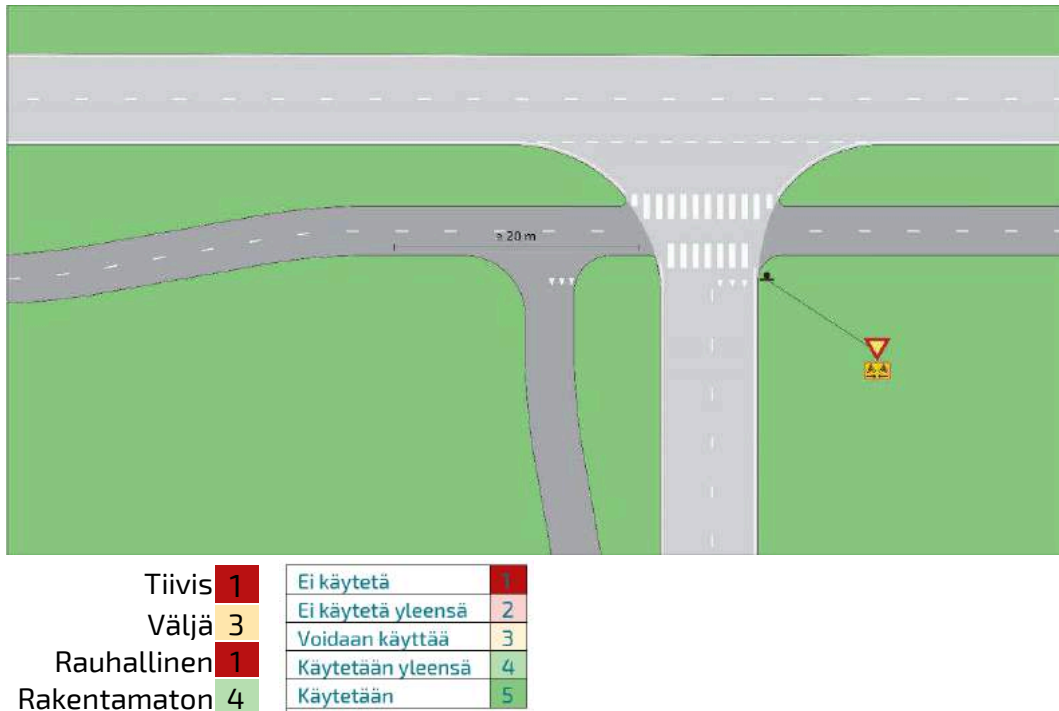
Kuva 145 Pääsuunnan pyörätie toteutetaan suoraksi 20 m ennen ajoradan ylitystä ja pyöräteiden keskinäinen risteys sijoitetaan riittävän etäälle ajoradan ylityksestä.
