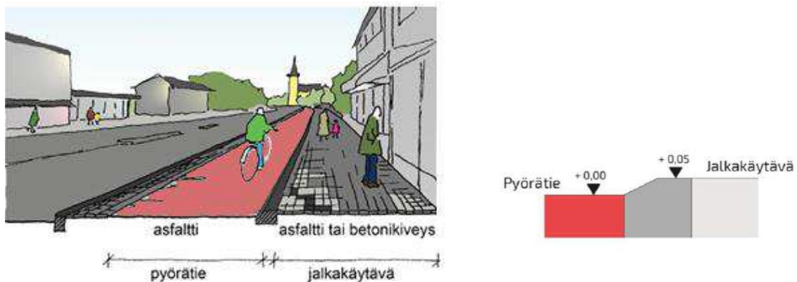
Kuva 32 Tasoerottelu (tasoero on yleensä välillä 0,05–0,08 m).
