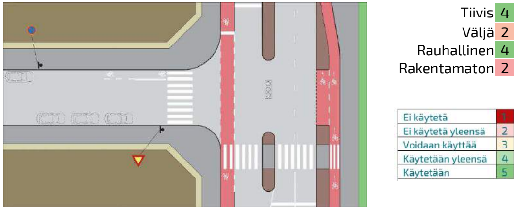
Kuva 123 Liikennevalo-ohjatussa risteyksessä vain pyöräliikenteelle sallitulle suunnalle merkitään yleensä pyöräkaista.
