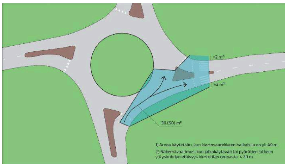
Kuva 98 Kiertoliittymän näkemät ajosuuntaan (mukaillen Tiehallinto 2001).
