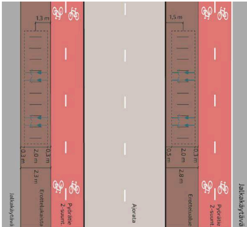
Kuva 187 Pyöräpysäköinti erottelukaistalla ja -alueella (kaaritelineet).
