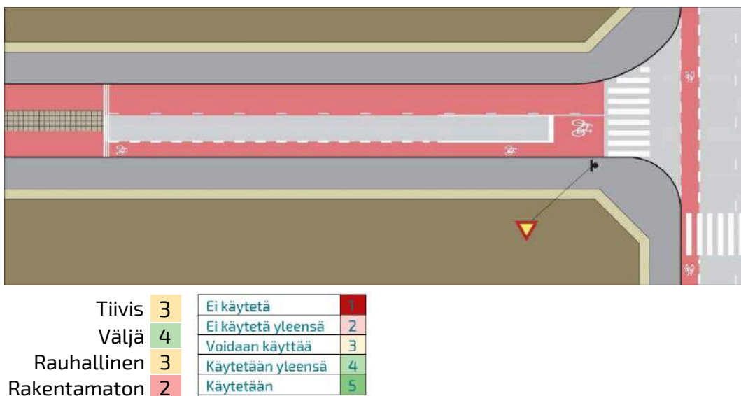
Kuva 131 Pyöräkadun päättävässä risteyksessä voidaan käyttää normaalia kapeampia ajokaistaleveyksiä.
