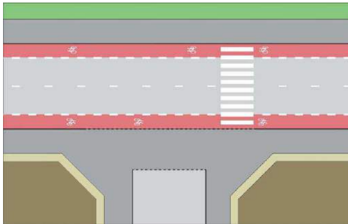
Kuva 105 Pyöräkaista rajautuu risteysalueella sivusuunnan yli jatkettuun rakenteeseen.
