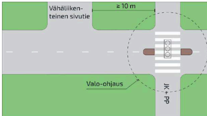
Kuva 168 Liikennevalo-ohjatun suojatien tai pyörätien jatkeen vähimmäisetäisyys liikennevalo-ohjaamattomasta kolmihaarisesta risteyksestä.
