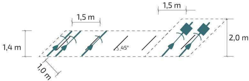
Kuva 180 Pyöräpysäköinnin tilantarve vinopysäköinnissä. Erikoispyörät sijoitetaan tarvittaessa pysäköintirivin päättyyn.
