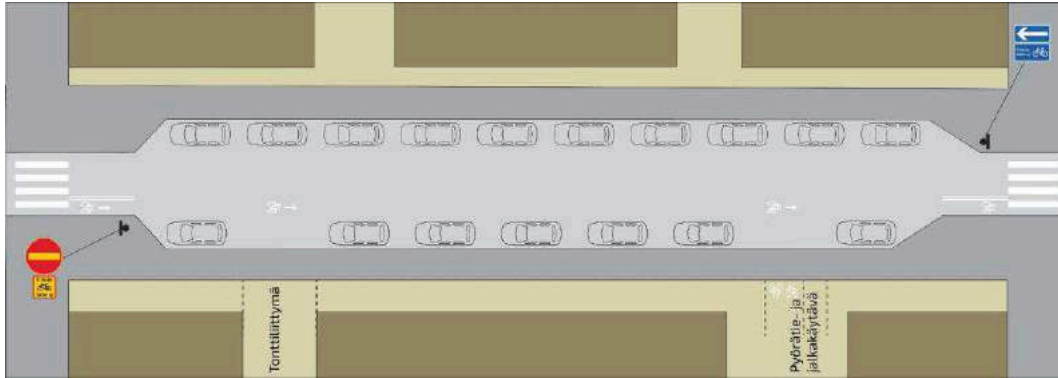
Kuva 40 Kaksisuuntainen pyöräliikenne yksisuuntaisella tiellä. Osuuden alkuun ja loppuun merkitään lyhyt pyöräkaista.
