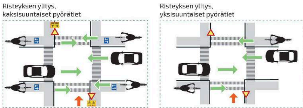
Kuva 8 Pyöräliikenteen ollessa kaksisuuntaista on risteyksissä runsaasti havainnointia edellyttäviä asioita. Kaksisuuntaisen pyörätien on todettu aiheuttavan turvallisuusongelmia risteämisissä.
