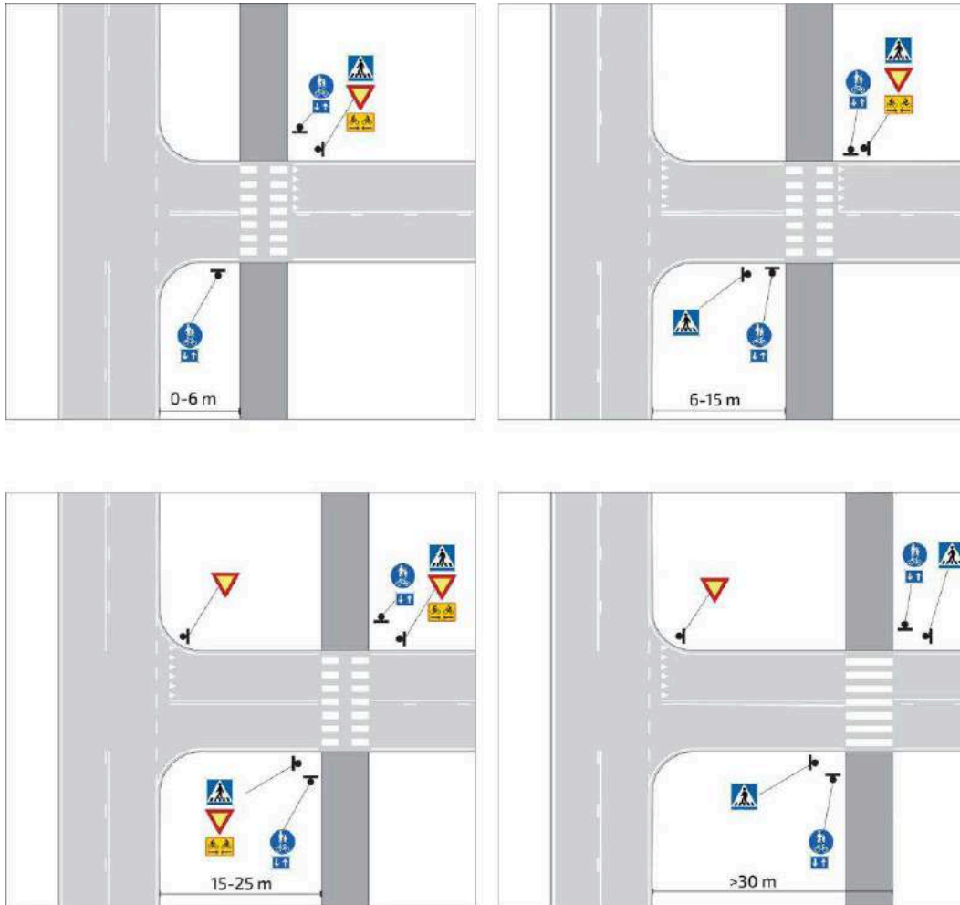
Kuva 92 Pyörätien ja ajoradan risteyskohdan väistämisvelvollisuuksien merkitseminen.
