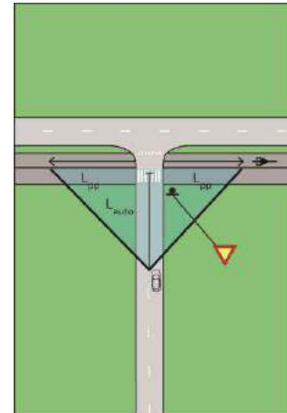
Taulukko 29 Näkemäalueet tasoliittymän yhteydessä olevassa pyörätien ja ajoradan risteyksessä, kun autoliikenne on väistämisvelvollinen. Pyöräliikenteen pääverkolla käytetään suositeltavia näkemäarvoja. Pyöräliikenteen ollessa väistämisvelvollinen sovelletaan taulukossa 28 olevan kuvan mukaisia L_{auto} arvoja.
