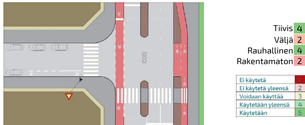
Kuva 124 Pyöräkaista varmistaa liikennevaloristeyksessä pyöräliikenteen pääsyn risteysalueelle ja osoittaa autoliikenteelle oikean ryhmittymiskohdan.
