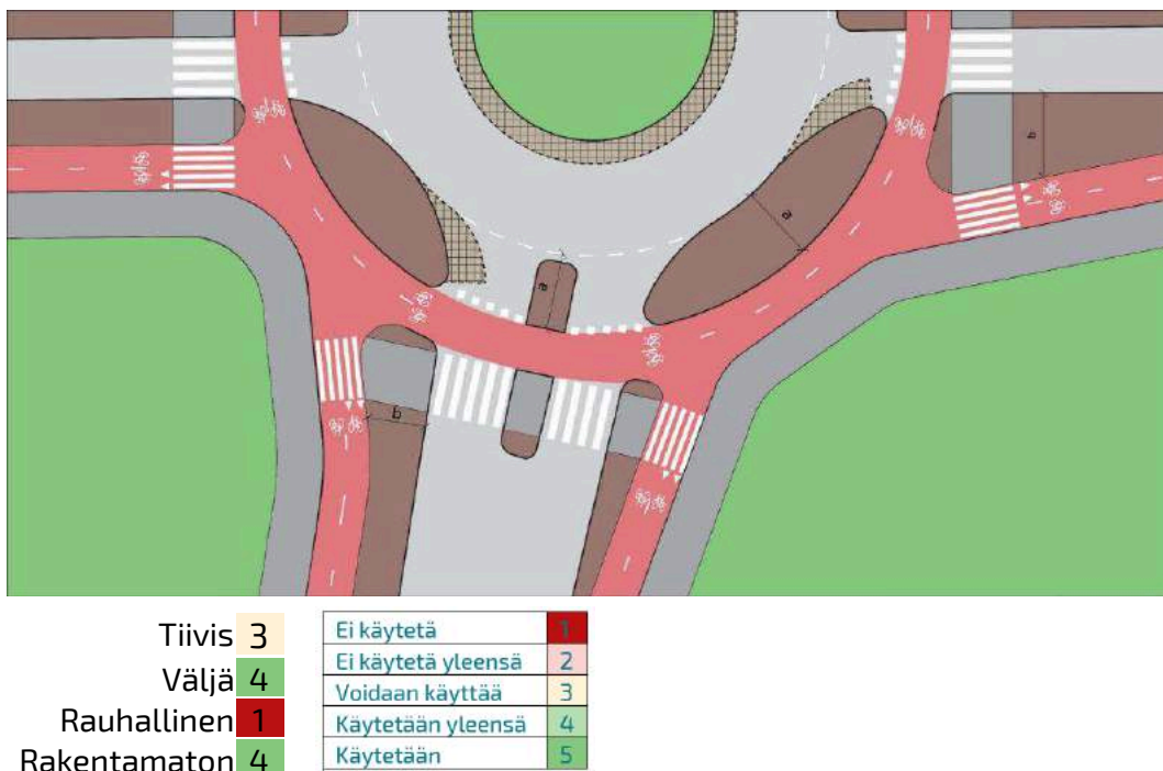
Kuva 148 Kaksisuuntainen pyörätie kiertoliittymässä.
