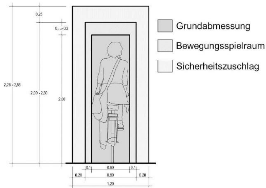
Abb. 29 Das Lichtraumprofil eines Velofahrenden bei Geradeausfahrt ( R > 80 m) und Steigung < 4 % gemäss VSS-Norm SN 640 201 [60]
